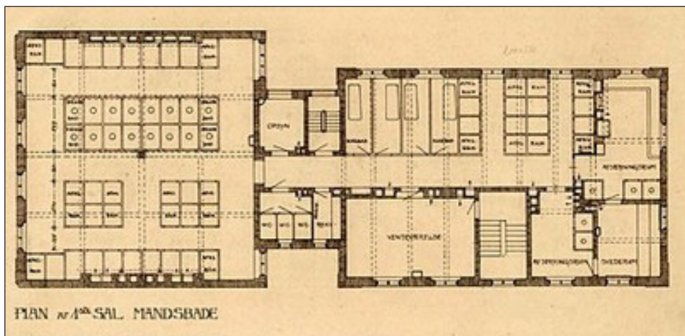
Plan af mandeafdelingen på 1. sal. (Stadsarkivets kort- og tegningssamling).
